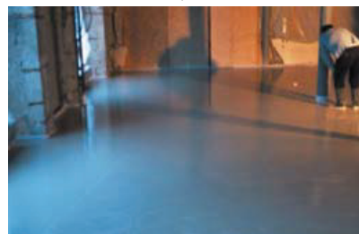
Berechnung Kabelabstand: m^2 : Kabellänge = Kabelabstand z.B. 20 m^2 : 110 m = 18,2 cm Abstand
